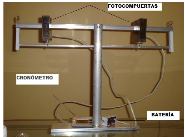
FIGURA 1. Prototipo del experimento.
