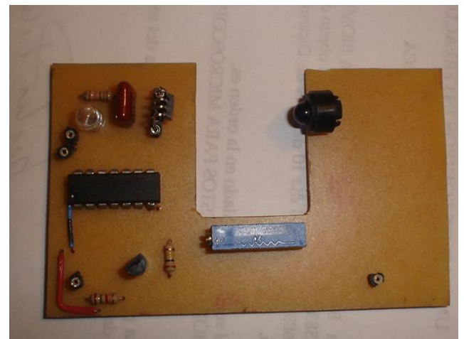
FIGURA 4. Compuerta y sus componentes.
