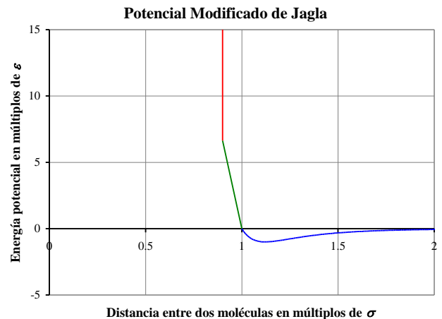
FIGURA 9. La gráfica muestra la forma final de la nueva aproximación del potencial de Lennard-Jones, la cual presenta tres zonas: una zona de potencial infinito que corresponde al intervalo 0 < r < \lambda , una zona positiva que se encuentra en el intervalo \lambda < r < \sigma y una zona negativa que corresponde al intervalo \sigma < r < +\infty .
