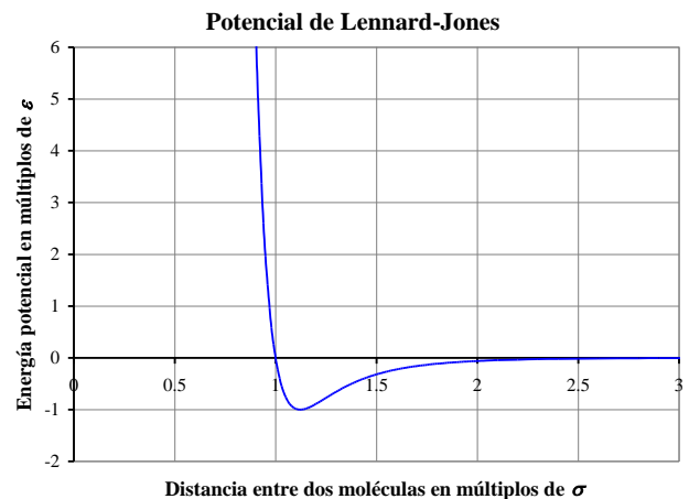
FIGURA 1. Gráfica del Potencial de Lennard-Jones realizada a partir de la ecuación (16). El eje horizontal corresponde a la distancia entre dos moléculas en múltiplos de \sigma y el eje vertical corresponde a la energía potencial de interacción entre dos moléculas en múltiplos de \epsilon .
